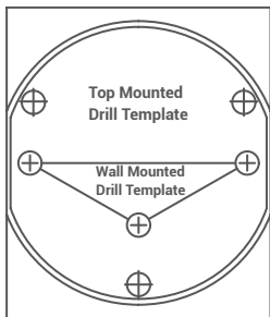
Vrtací šablona (1×)
