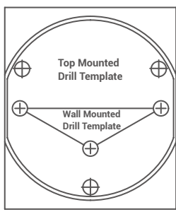
Vrtací šablona (1×)
